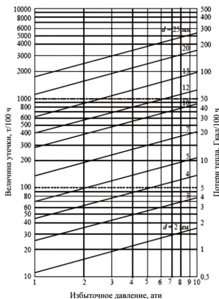
Рис. 1. Номограмма для определения величины утечки сетевой воды и потерь тепла (при T_v = 55 °С).
