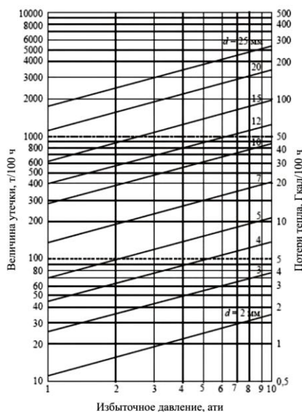
Рис. 1. Номограмма для определения величины утечки сетевой воды и потерь тепла (при T_{в} = 55 \text{ }^{\circ}\text{C} ).
