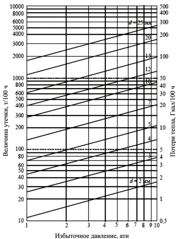
Рис. 1. Номограмма для определения величины утечки сетевой воды и потерь тепла (при T_v = 55 \text{ }^\circ\text{C} ).
