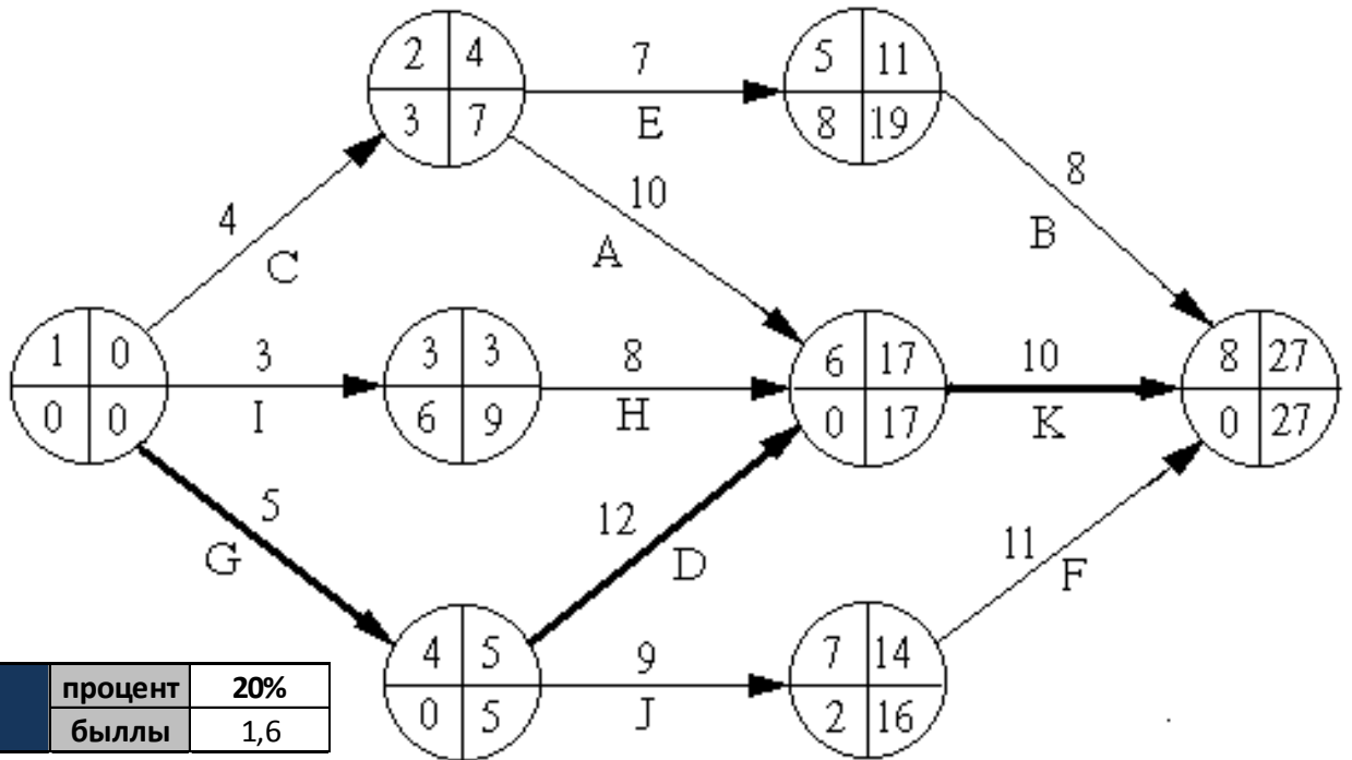
Рис.1. Сетевая модель
