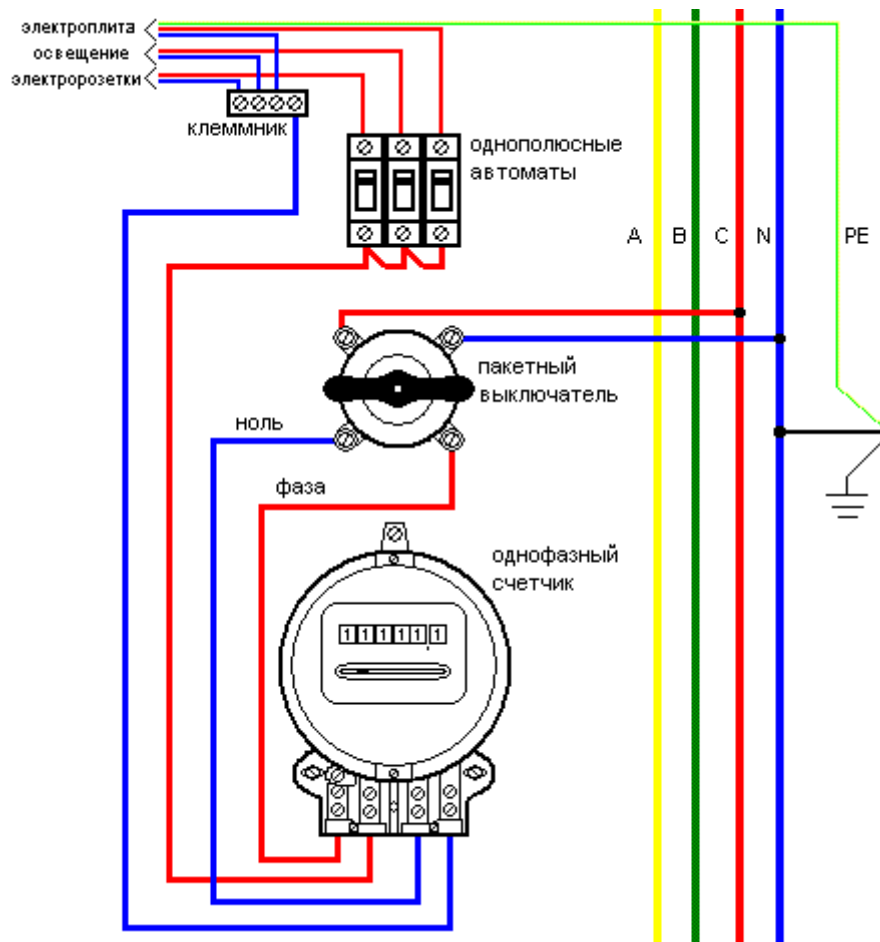
Рис.2 Электрический счетчик
